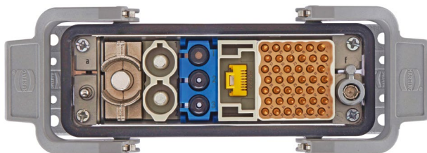
Złącze modułarne systemu Han-Modular z możliwością dostosowania pod indywidualne potrzeby każdej aplikacji
