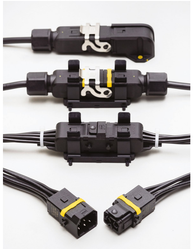
Złącza serii Han 1A
