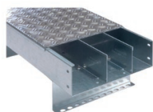
KORYTA KABLOWE
